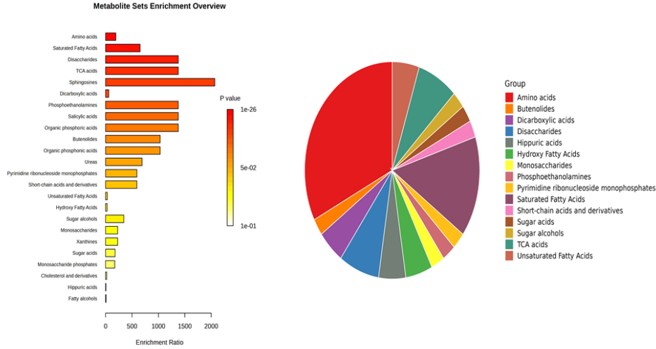
Şekil 3: Metabolit sınıflandırması
